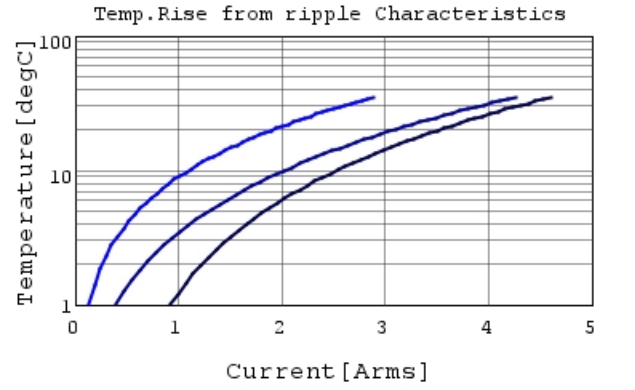
GRM21BR71C475KA73 Temp.rise — 100kHz
