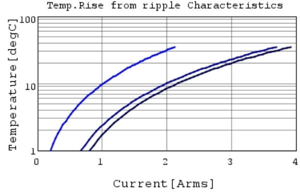
GRM21BR71E225KA73 Temp.rise — 100kHz
