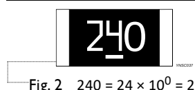
Fig. 2 240 = 24 \times 10^0 = 24
