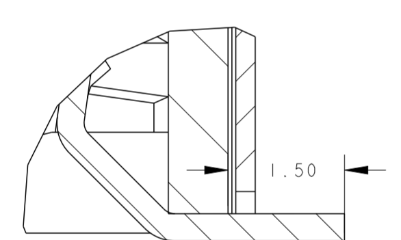
DETAIL Z SCALE 15:1
